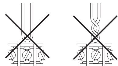
Figura 15: Conexión incorrecta
