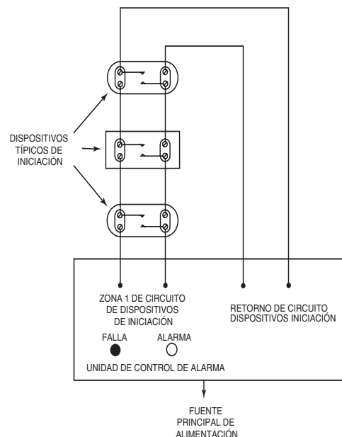
Figura 11: Detectores bifilares, circuito Estilo D (Clase A)
