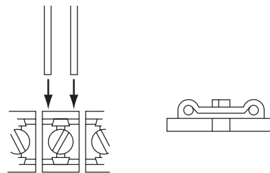
Figura 14: Conexión correcta
