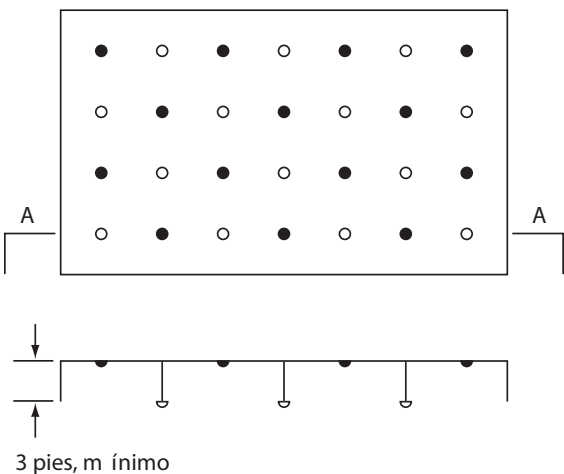
Figura 22: Separación de detectores en techos inclinados (a dos aguas)
